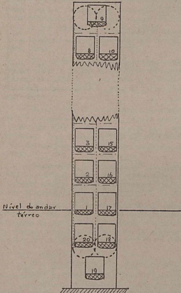
Fig. 34 - Uma unidade do sistema mecânico, para alojamento vertical.
