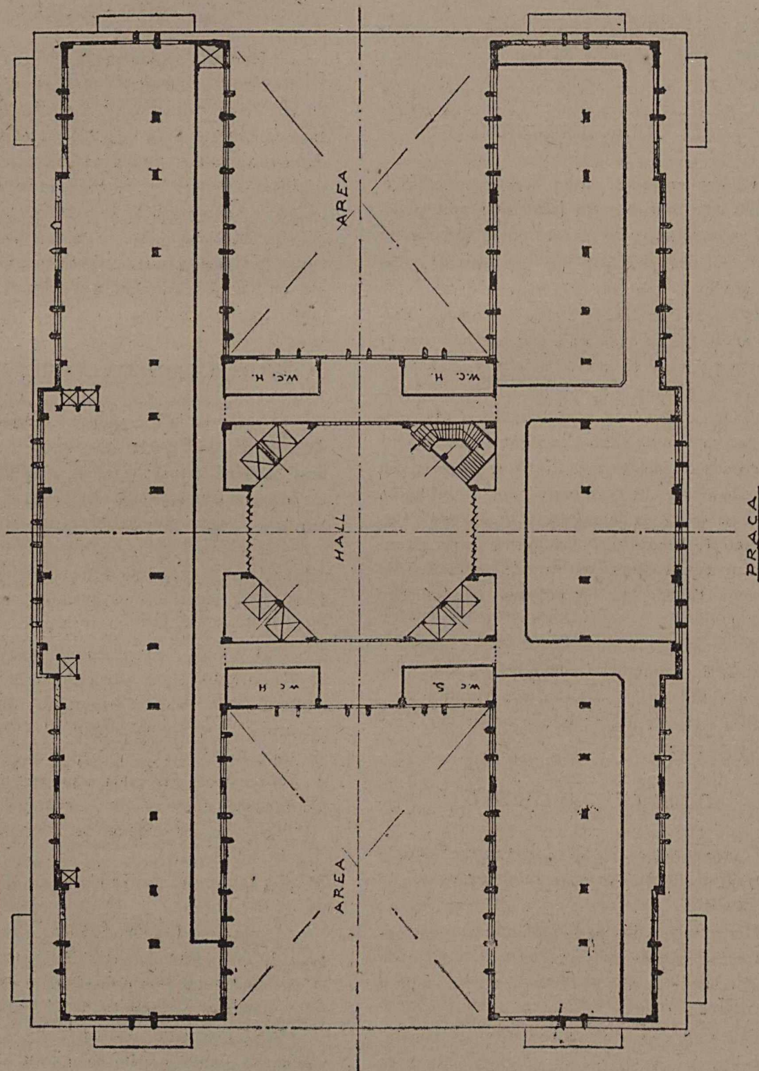
PLANTA DO ANDAR TIPO
